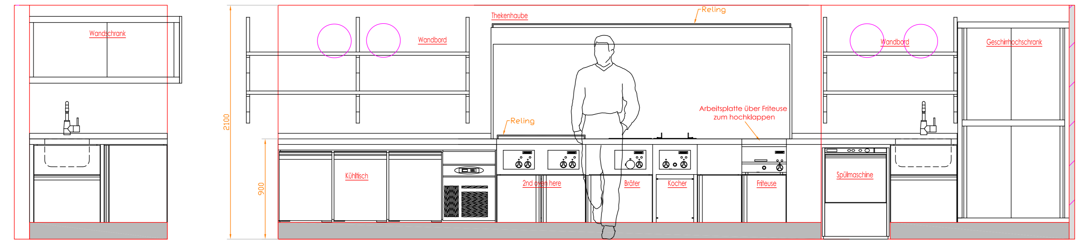
Vorderansicht Kochzeile - Spülen
